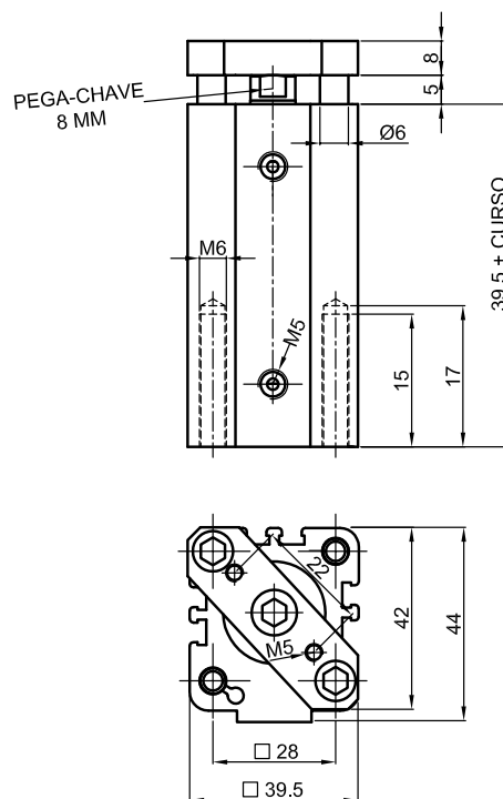
Cilindro com Antigo Ø 40
