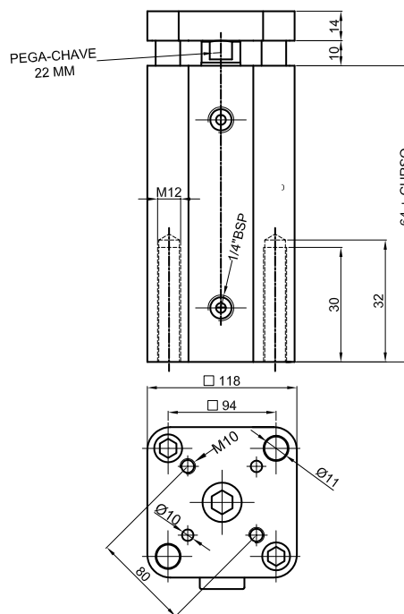
Cilindro com Antigo Ø 100
