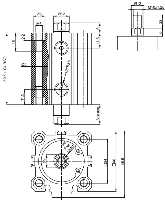
Cilindro com Haste Passante Ø 32
